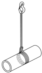
Figure C.1 — Élingage bagué double
