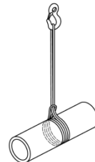
Figure C.1 — Élingage bagué double
