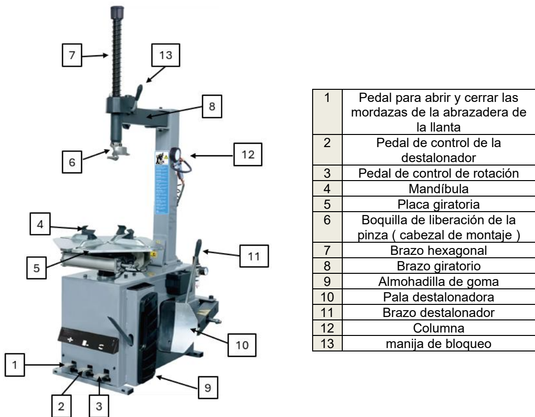
Figura 2-3 Color de la máquina no contractual
