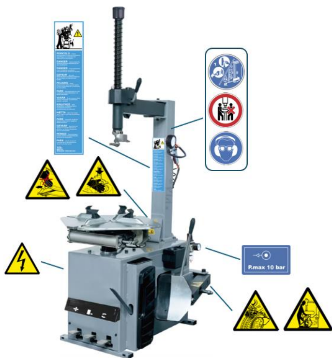
Figura 1-3 Color de la máquina no contractual
