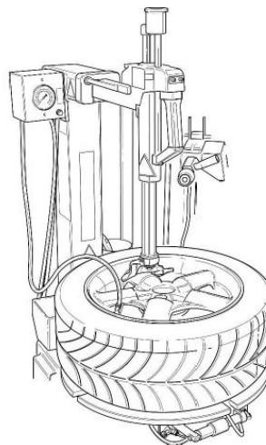
Fig. 4-4-1 Serrage de la roue avec l'outil
